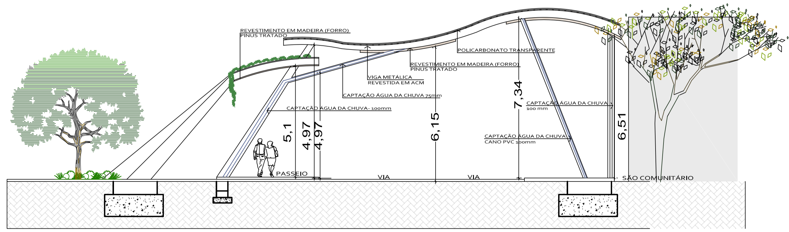
CORTE BB
